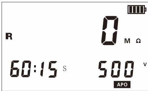
图 9-1 吸收比模式 15 秒模式
